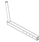
Guide Pole (4)
